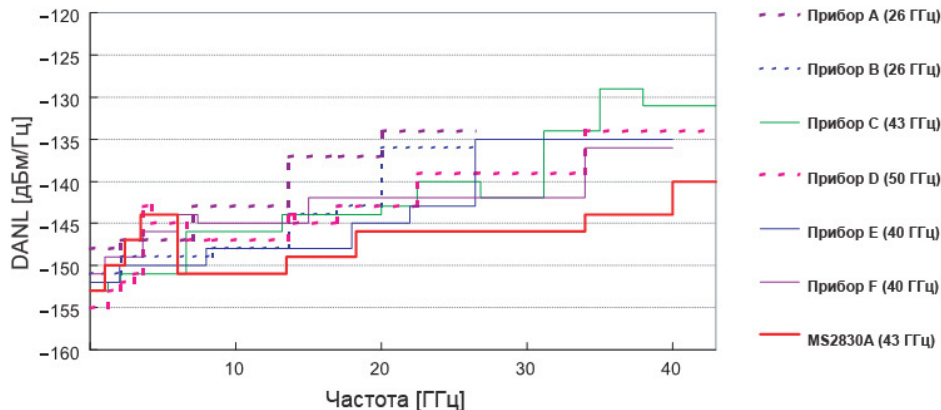
Сравнение характеристик приборов по среднему отображаемому уровню шума (DANL)
